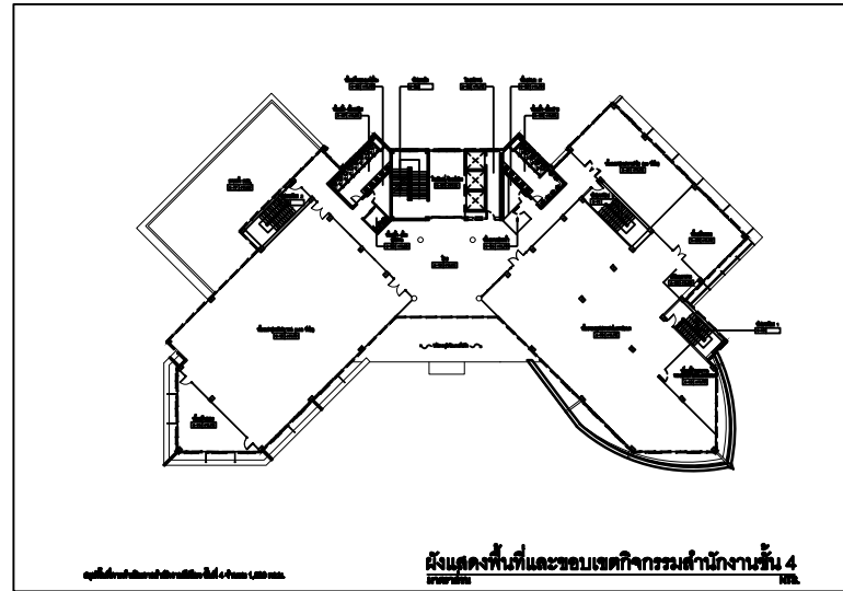
ผังบริเวณและแปลนพื้นที่ชั้น 4 มาตรฐาน NTS.
