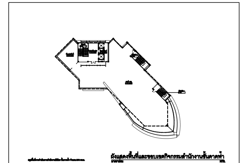
ผังบริเวณและแปลนพื้นที่ชั้นดาดฟ้า มาตรฐาน NTS.
