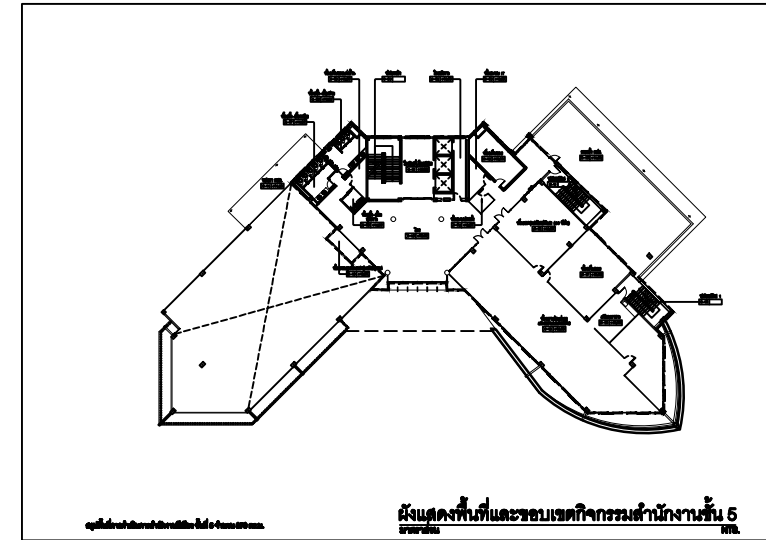
ผังบริเวณและแปลนพื้นที่ชั้น 5 มาตรฐาน NTS.
