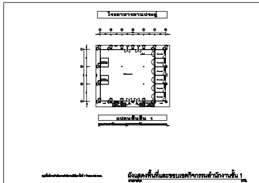
ผังบริเวณและแปลนพื้นที่ชั้น 1 มาตราส่วน NTS.
